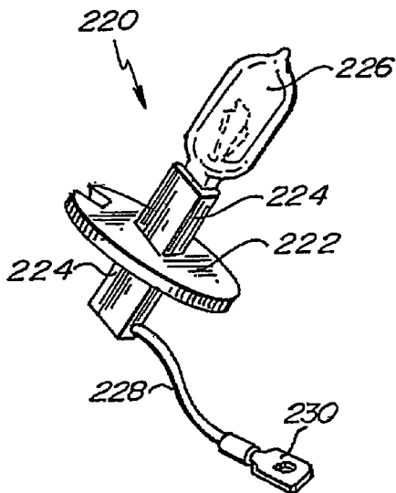
Fig. 18. PRIOR ART
