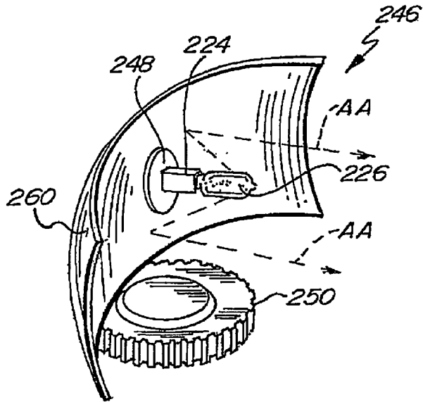
Fig. 20. PRIOR ART
